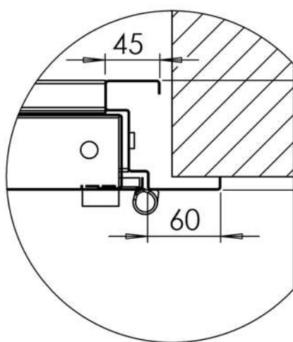
Рис. 1 Угловая рама
