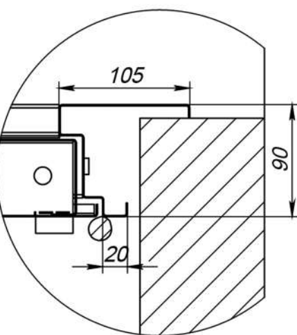
Рис. 3 Угловая рама (обратная)
