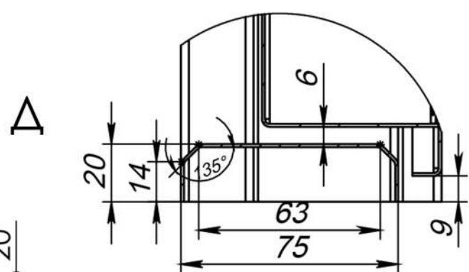
Рис. 6 Накатной порог
