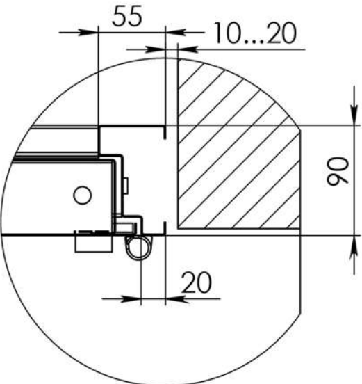
Рис. 4 Торцевая рама
