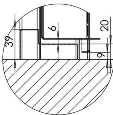
Рис. 5 Высокий порог
