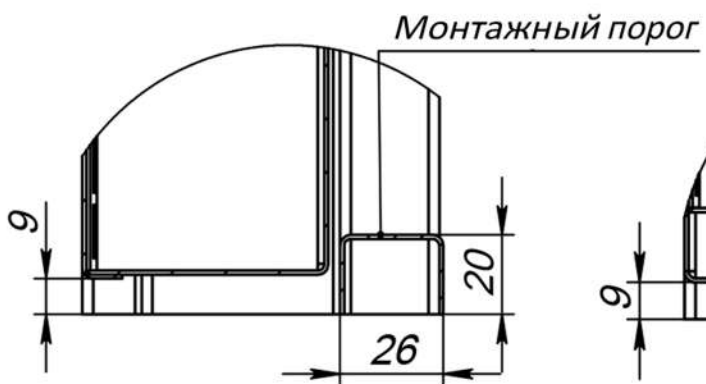
Рис. 8 Без порога
