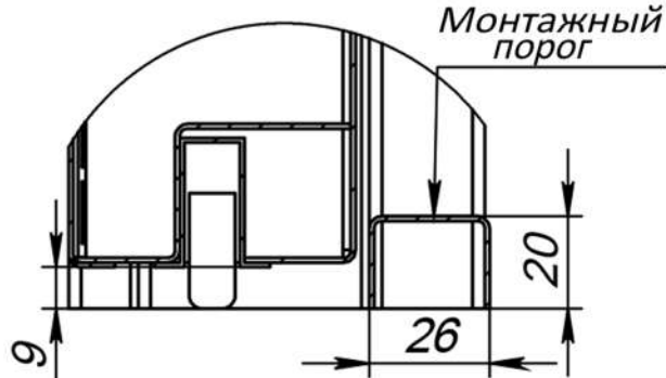
Рис. 7 Автоматический порог
