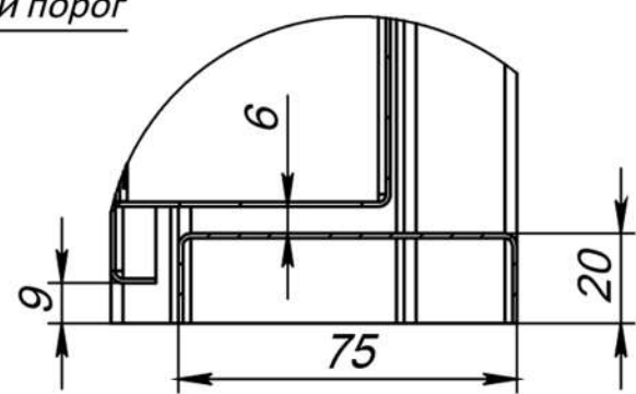
Рис. 9 Низкий порог
