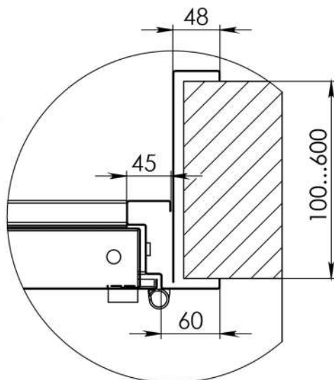
Рис. 2 Угловая рама (в обхват)
